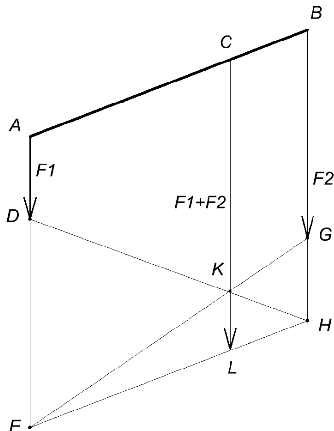
Рисунок 3. Определение точки приложения равнодействующей силы.
