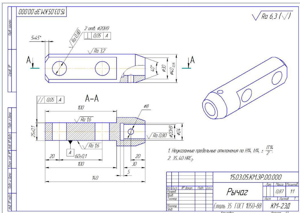
Рисунок 2 – Чертёж детали, созданный на основе 3D-модели
