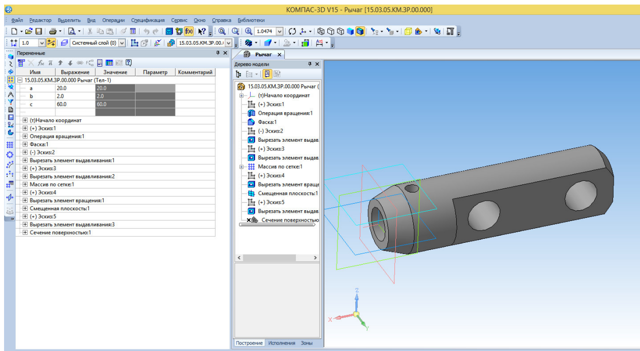
Рисунок 1 – 3D-модель детали с таблицей переменных
