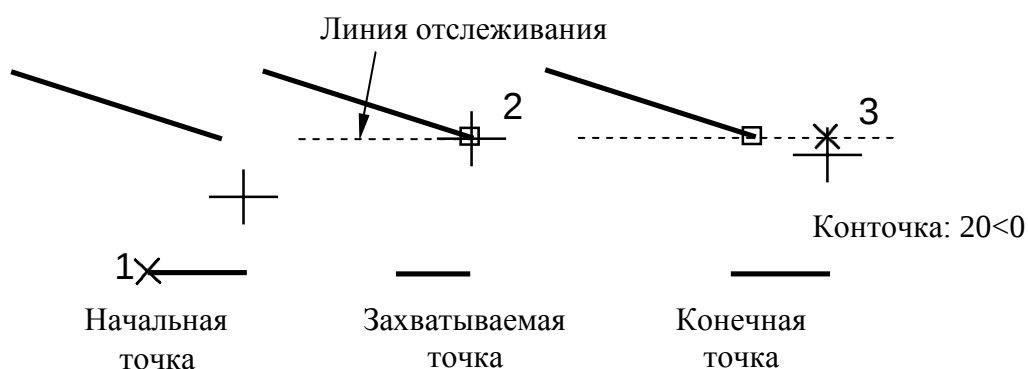
Рисунок 10 – Объектное отслеживание
