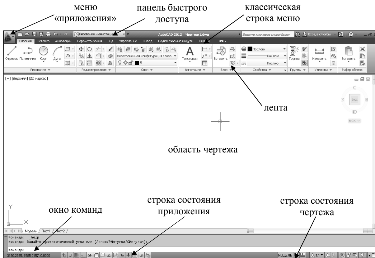
Рисунок 1 – Интерфейс AutoCad 2012
