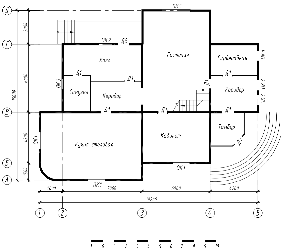
Рисунок 34 – Схема здания
