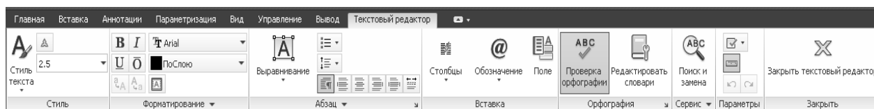
Рисунок 14 – Текстовый редактор
