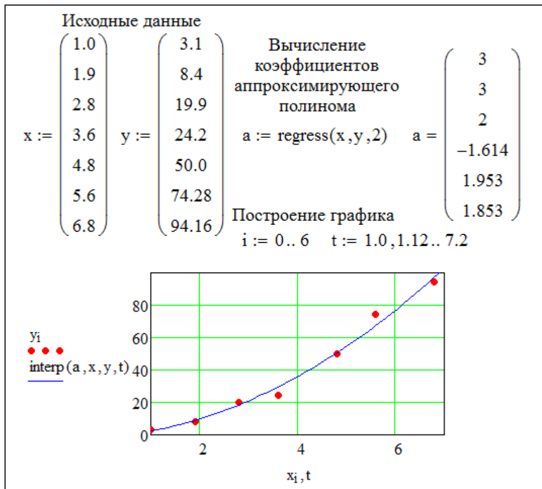
Рисунок 4.4 - Аппроксимация данных полиномом второго порядка
