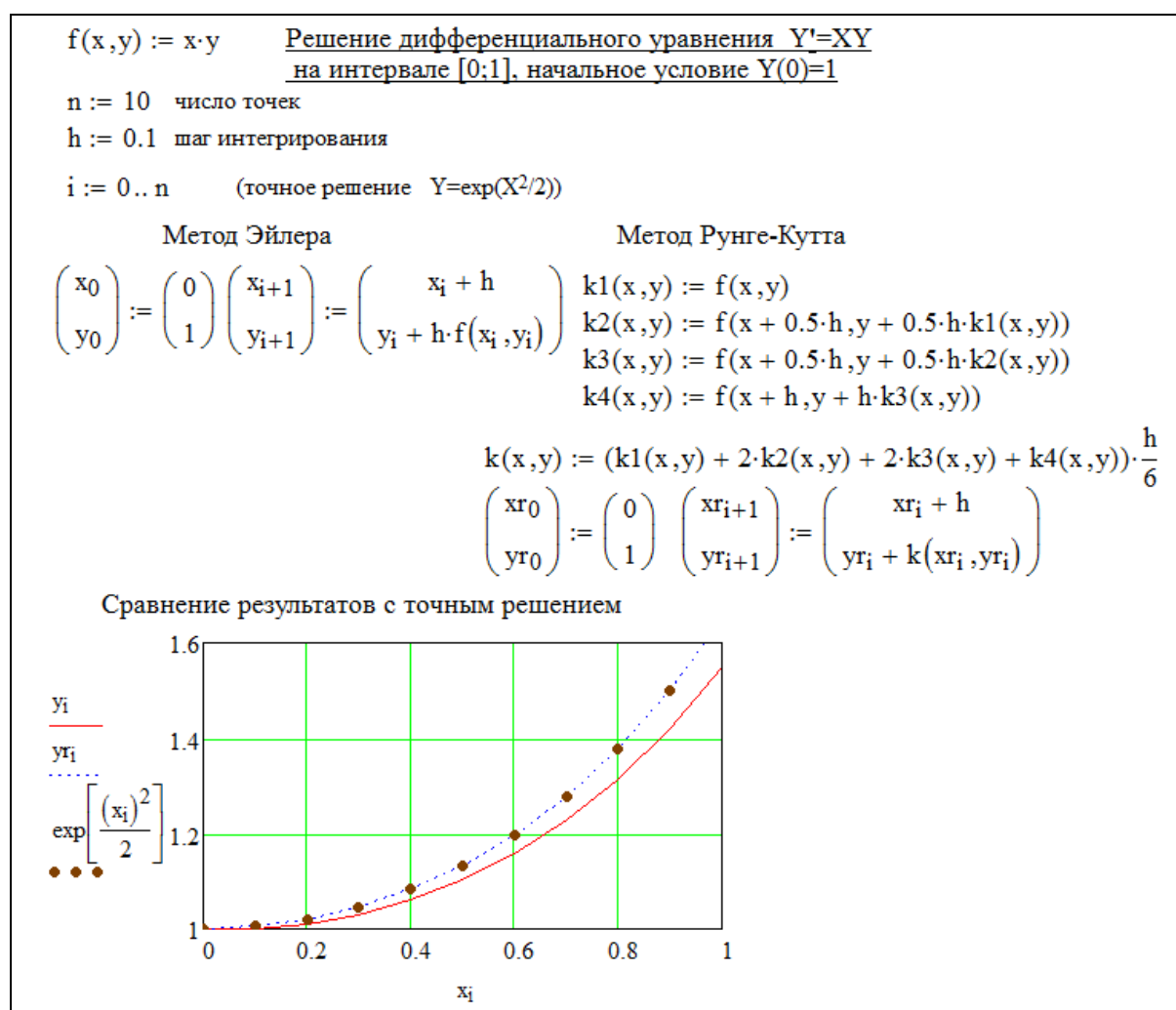
Рисунок 5.1 - Решение дифференциального уравнения методами Эйлера и Рунге-Кутты
