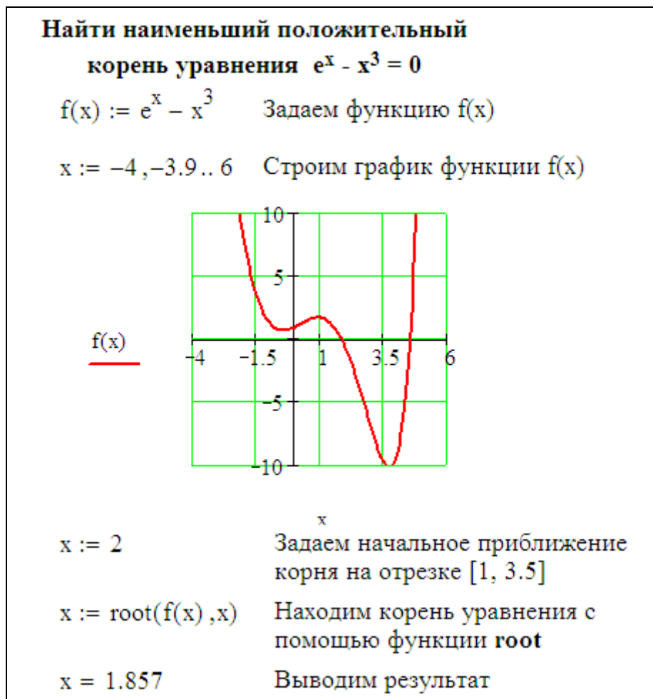
Рисунок 1.1 – Пример использования функции root
