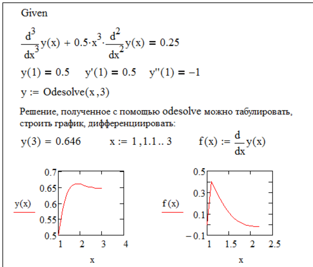
Рисунок 5.7 - Решение дифференциального уравнения третьего порядка с помощью odesolve
