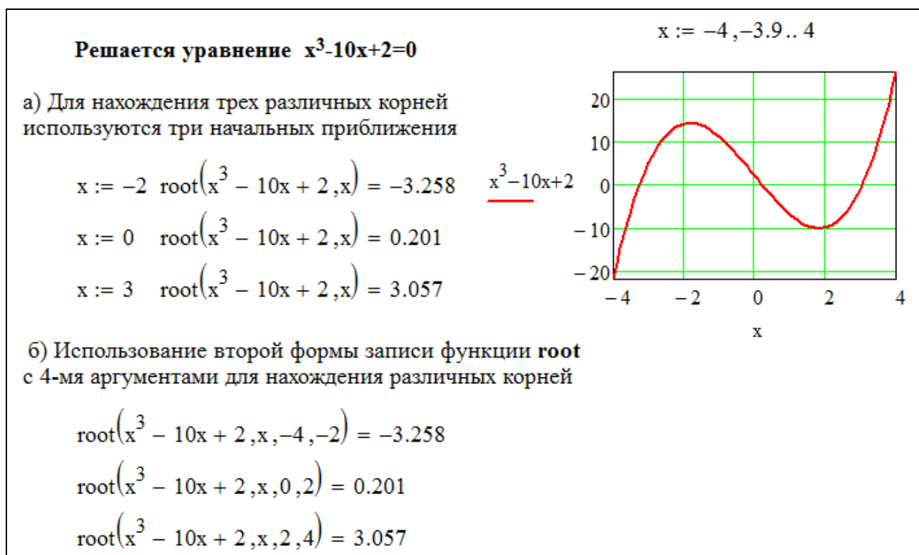
Рисунок 1.2 - Использование функции root для нахождения корней уравнения
