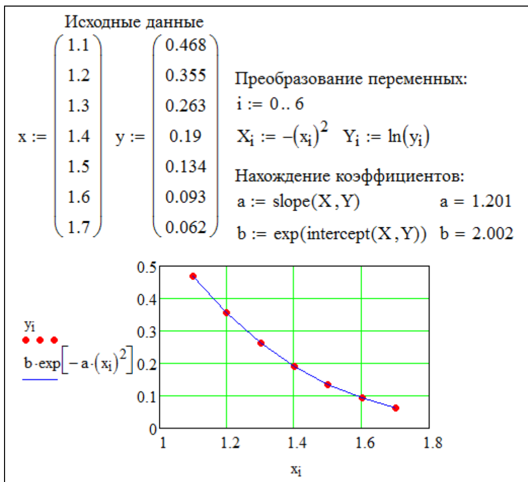
Рисунок.4.2 - Аппроксимация данных зависимостью y = b \cdot \exp(-a \cdot x^2)
