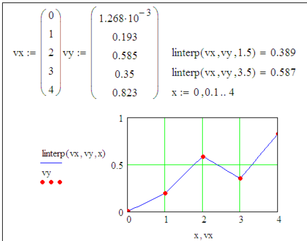
Рисунок 3.1 - Примеры линейной интерполяции
