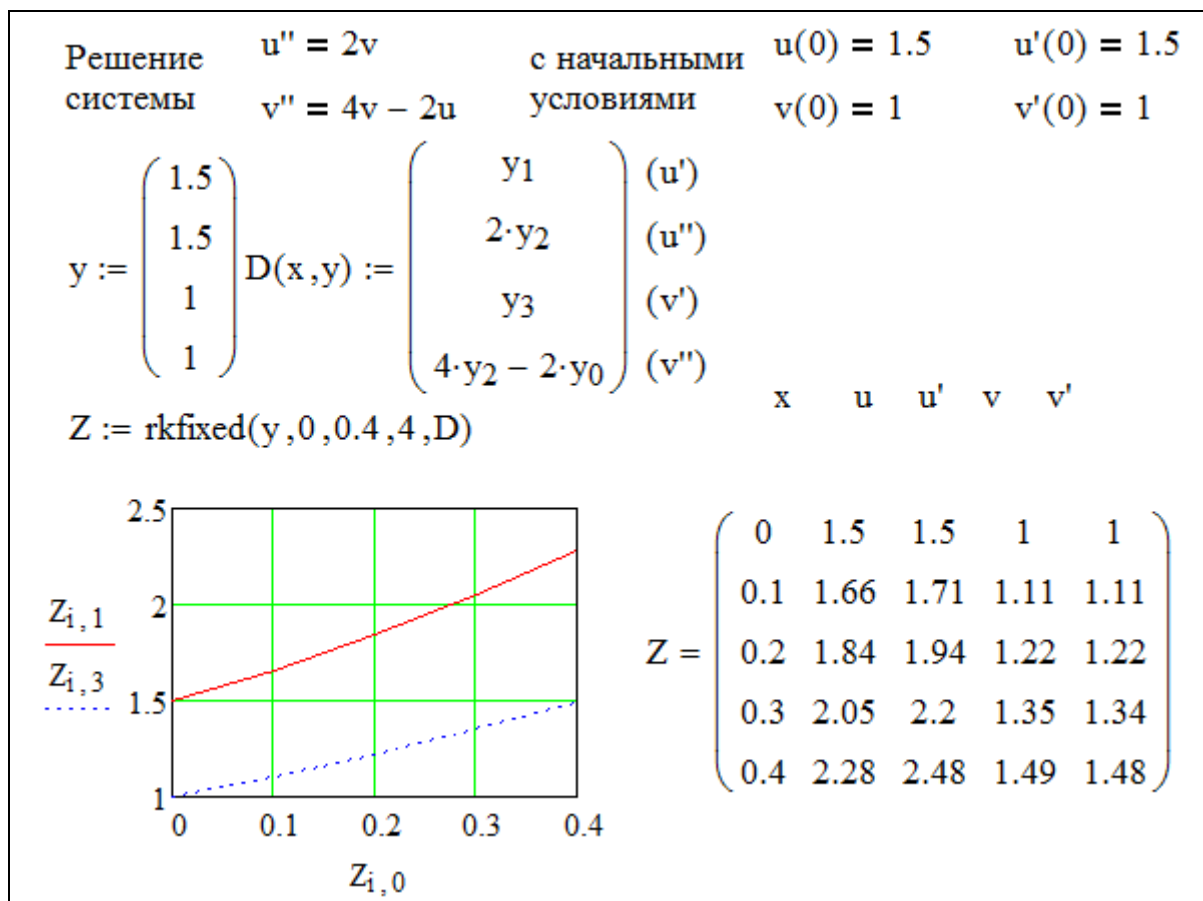
Рисунок 5.5 - Решение системы дифференциальных уравнений второго порядка
