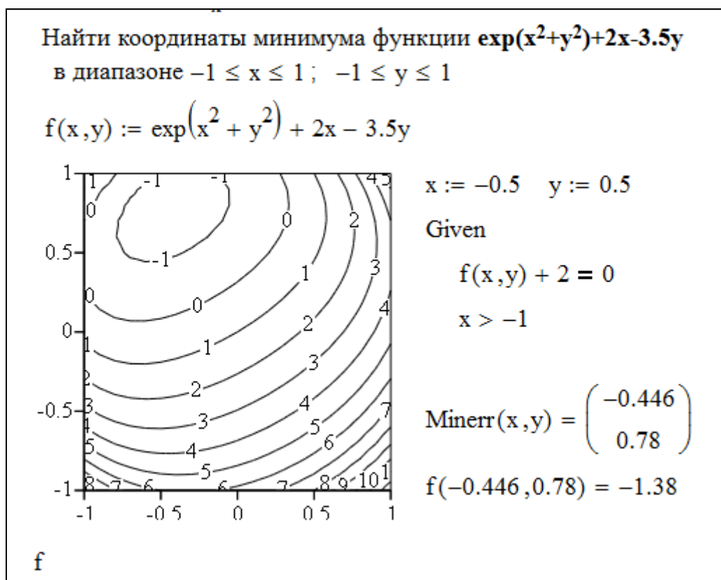
Рисунок 2.3 - Пример нахождения минимума функции двух переменных
