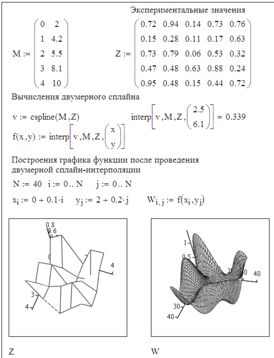
Рисунок 3.4 - Пример двумерной интерполяции кубическим сплайном
