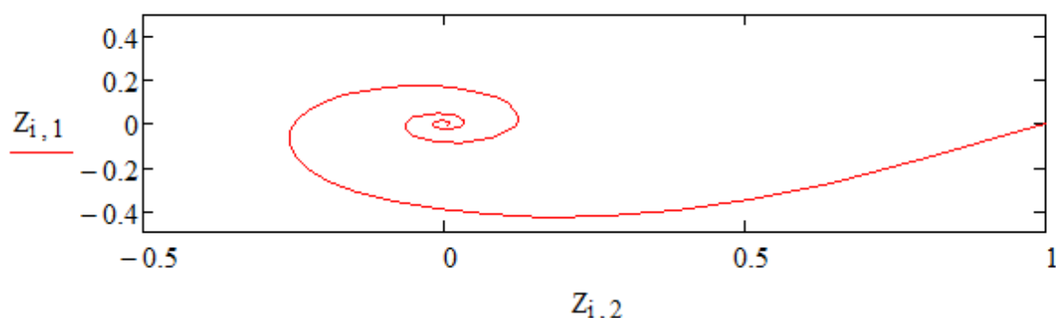
Рисунок 5.3 - Решение системы двух дифференциальных уравнений первого порядка
