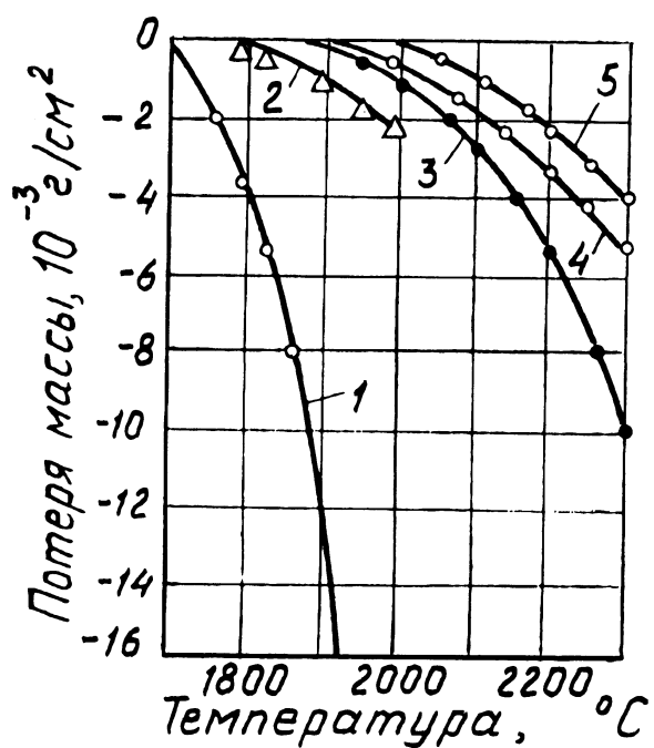
Рисунок 12 - Зависимость потери массы оксидных керамик в вакууме ( P = 0,013 Па) от температуры
