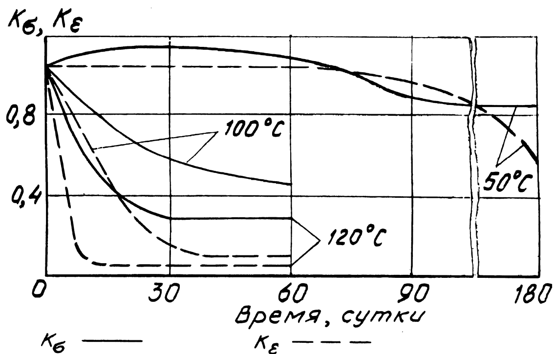
Рисунок 13 - Коэффициенты изменения механических свойств капрона K_\sigma и K_\epsilon в процессе старения при различных температурах
