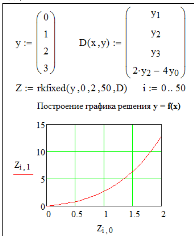
Рисунок 5.4 - Решение дифференциального уравнения четвертого порядка
