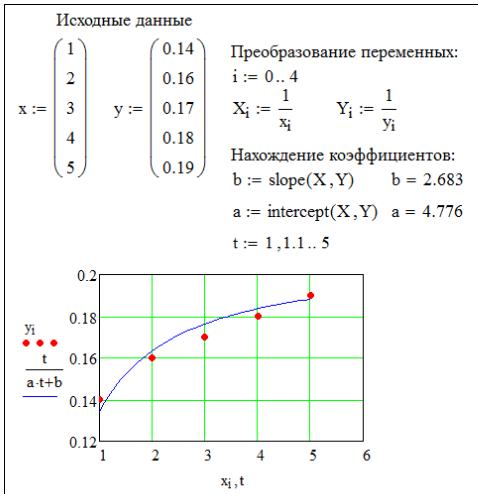
Рисунок.4.3 - Аппроксимация данных зависимостью y = x/(a \cdot x + b)
