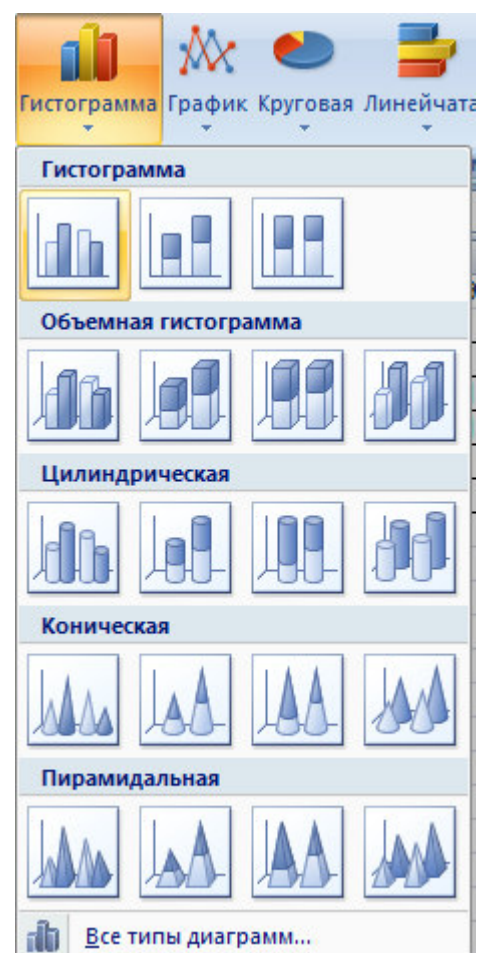
Рисунок 1.5 – Виды гистограмм
