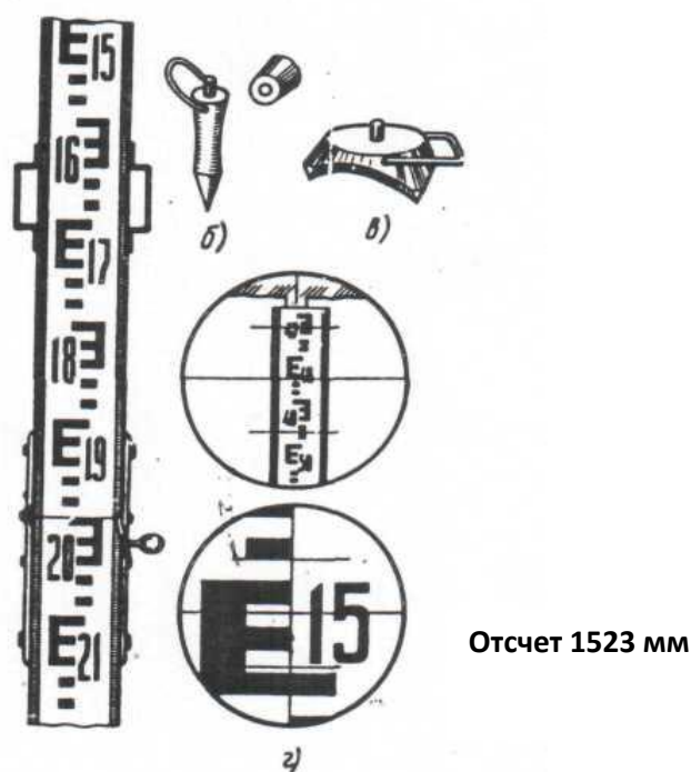
Рисунок 16 - Нивелирные рейки
