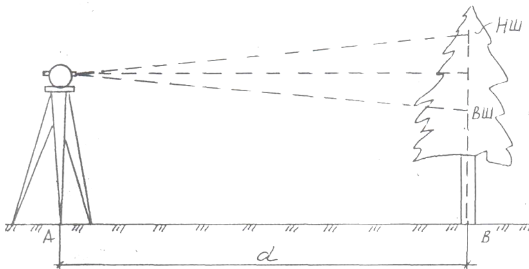
Рисунок 2 Схема измерения расстояний дальномером
