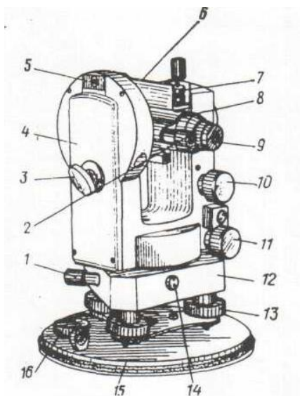
Рисунок 4 - Общий вид теодолита 2Т 30
