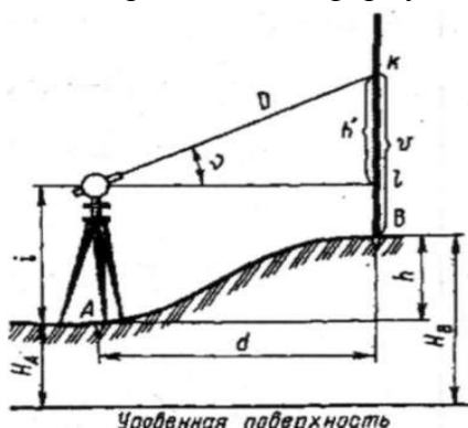
Рисунок 20 Тригонометрическое нивелирование
