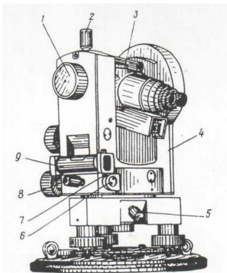
Рисунок 3 - Теодолит 2Т 30
