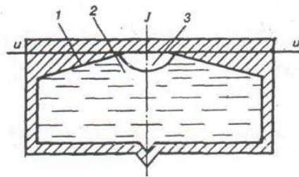
Рисунок 14 - круглый уровень 1-ампула, 2- жидкость, 3- пузырек.
