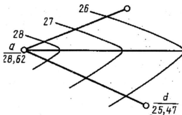
Рисунок 22 Горизонтали
