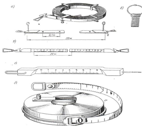
Рисунок 1 Приборы для линейных измерений
