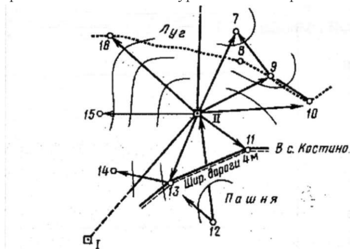
Рисунок 21 Абрис тахеометрической съёмки
