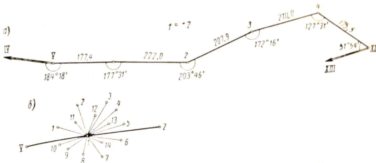
Рисунок 25 а)- тахеометрический ход; б)-съемка с пункта тахеометрического хода.
