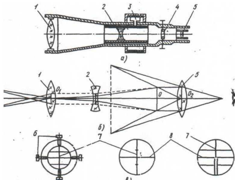
Рисунок 12 - Зрительная труба (разрез а), оптическая схема (б) и поле зрения и сетки нитей в различных приборах (в); 1- объектив, 2- линза, 3-трибка, 4- стеклянная пластинка, 5- окуляр, 6- регулировочные винты, 7,8- вертикальные и горизонтальные нити.
