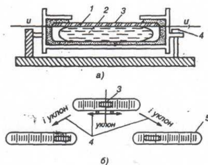
Рисунок 13. Цилиндрический уровень и уклоны при положении пузырька. а) вид с боку, б) вид сверху; 1- ампула; 2- жидкость; 3- пузырек; 4- исправительный винт; 5- уклон ампулы.
