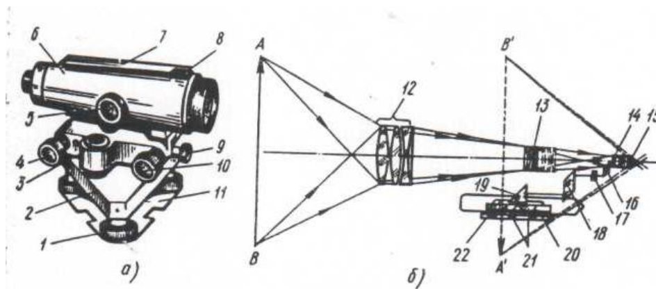
Рисунок 15 - Нивелир Н-3 (а) и его оптическая схема (б)
