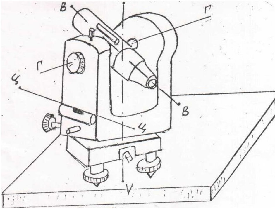
Рисунок 8 Основные оси теодолитов
