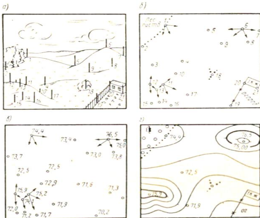
Рисунок 23 а)- расположение речных точек; б)- кроки; в) план в отметках; г)- в горизонталях
