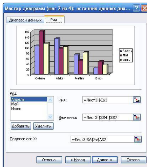
Рисунок 7.6 – Вкладка Ряд
