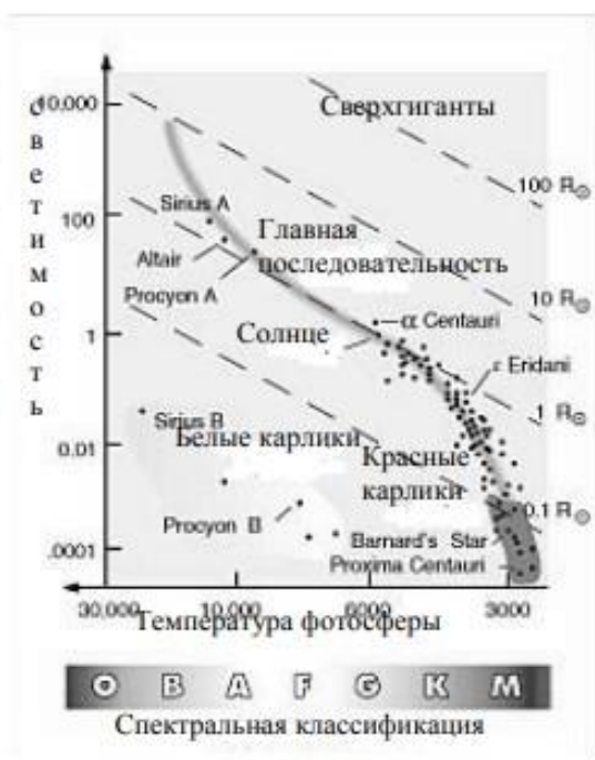
Рис.14 Диаграмма Герцшпрунга-Рассела
