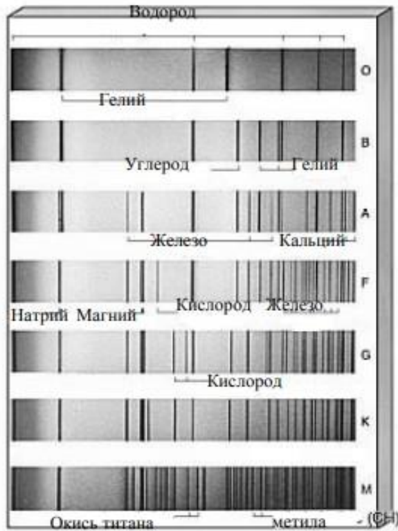
Рис. 13 Спектры
