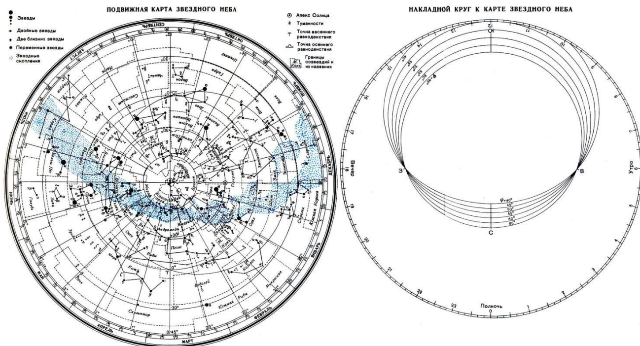
Рисунок 1 - Звездная карта
